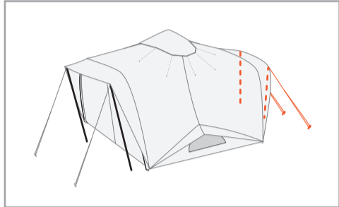
반대쪽도 똑같이 반복해서 지주 폴대와 라운딩 폴대를 넣어주세요.
