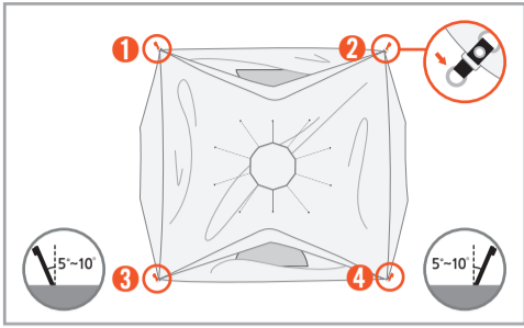
그라운드시트를 펼치고 그 위에 본체 스킨을 펼쳐주세요. 모서리 4곳 아래쪽 O링에 껍다운 해주세요.
