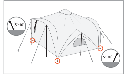
모서리의 처마 끝부분 4곳에 껍다운 해주세요.
