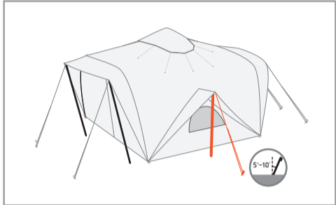
측면 지주 폴대를 세우기 위해 1곳에 껍다운 하고, 스트링을 이용해서 지주 폴대를 세워주세요. (좌/우 동일)
