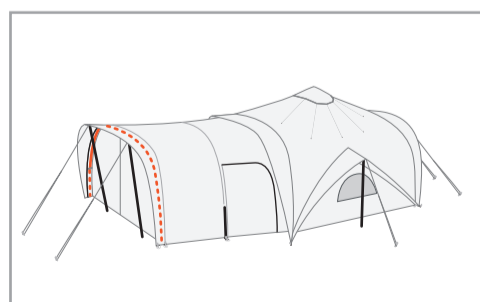
베스티블 출입문 메인 폴대를 체결해 주세요.
