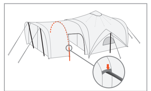
베스티블 중간에 중간 폴대를 끼워주세요.
