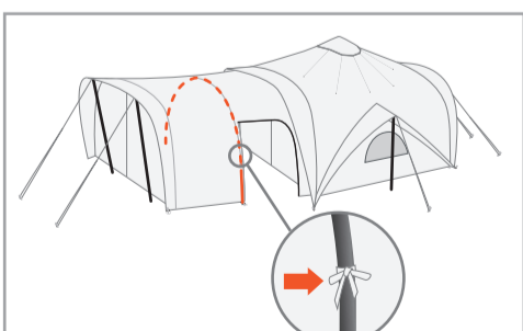
베스티블 중간 폴대를 세워서 반대쪽 아일릿에 체결해 주세요. 안쪽 실링 부분 폴대를 리본으로 묶어주세요.
