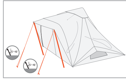
지주 폴대를 세우기 위해 2곳에 껍다운 하고, 스트링을 이용해서 지주 폴대를 세워주세요.
